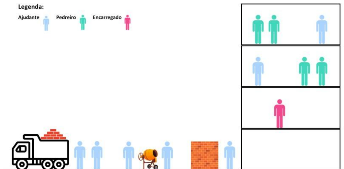
Figura 4 – Esquema Global de Execução de Alvenaria
