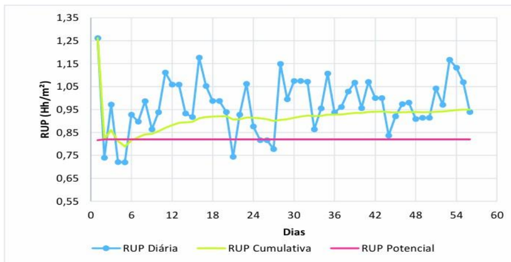
Figura 9 – Valores de RUP Diária, RUP Cumulativa e RUP Potencial para a Equipe A
