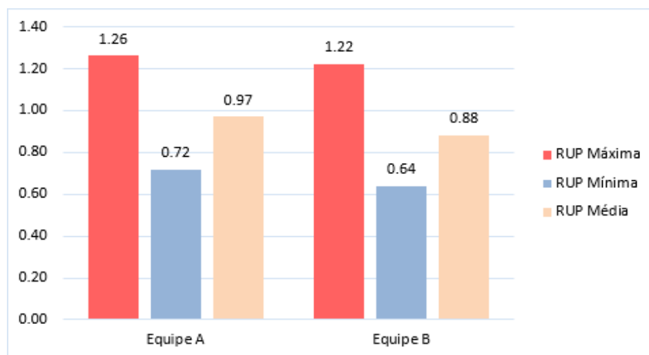
Figura 11 – Comparativo para a RUP Diária de cada equipe
