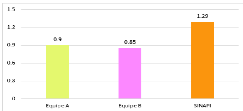
Figura 14 – Comparativo da RUP Cumulativa em relação ao SINAPI
