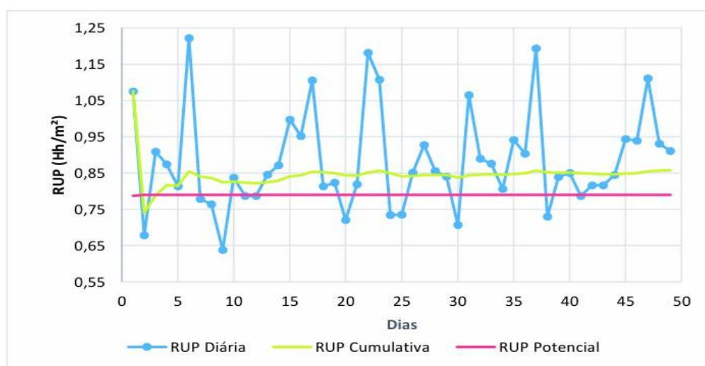
Figura 10 – Valores de RUP Diária, RUP Cumulativa e RUP Potencial para a Equipe B
