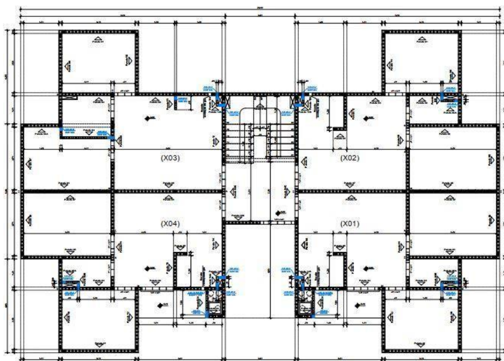
Figura 8 – Modelo de planta baixa de primeira fiada do pavimento tipo
