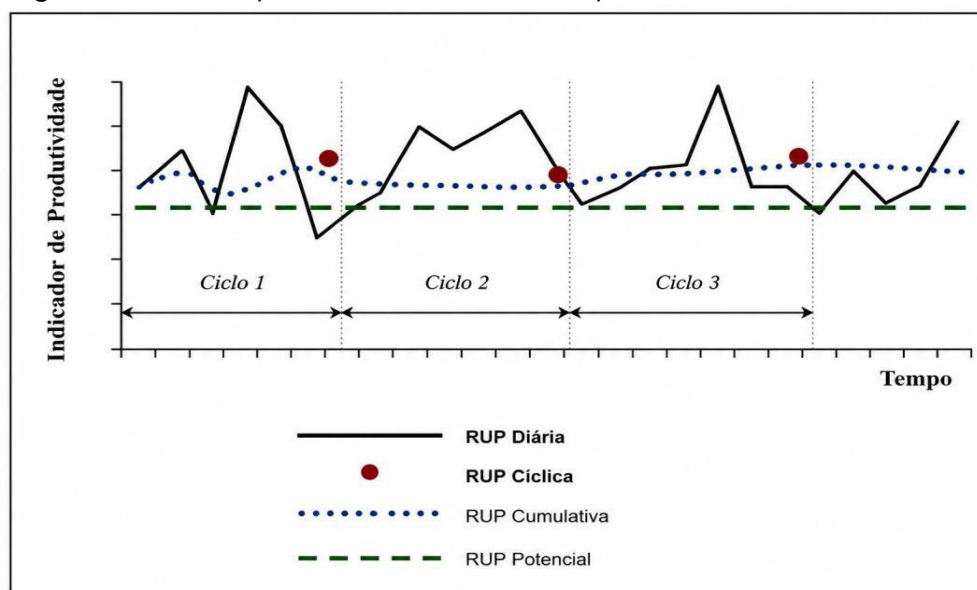
Figura 3 – Gráfico representativo dos diferentes tipos de RUP
